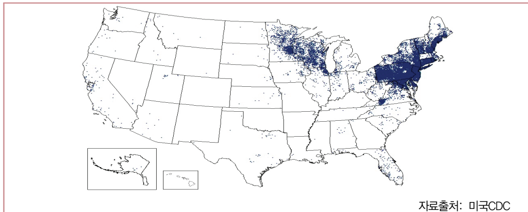
[그림 22] 미국의 라임병 발생현황(2016)
