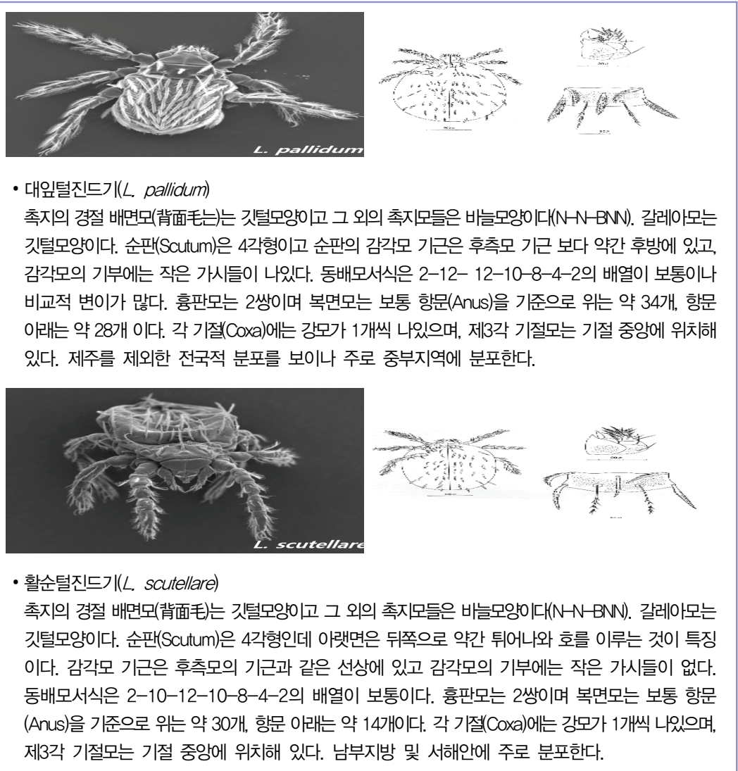
[그림 24] 주요 매개종의 형태적 특징
