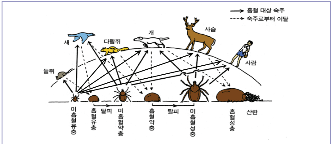
[그림 30] 숙주 진드기의 생활사 56)
