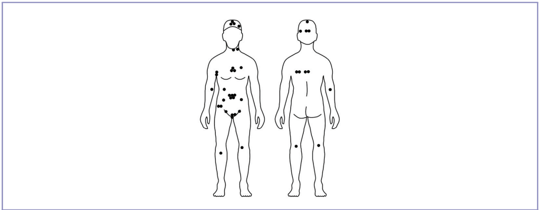
[그림 28] 참진드기 주요 인체 흡혈부위 55)
