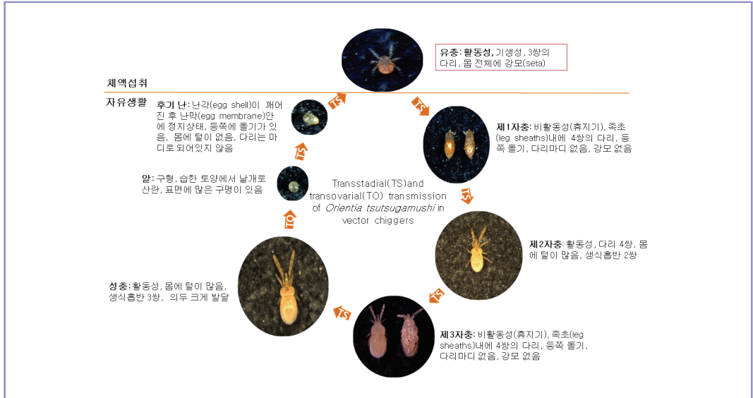
[그림 26] 대잎털진드기의 생활사
