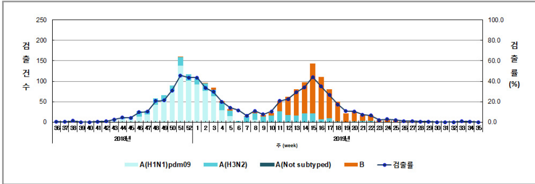
[그림] 2018-2019절기 인플루엔자 바이러스 검출현황 ※ 2018년 36주 ~ 2019년 35주 (2018. 9. 2. ~ 2019. 8. 31)
