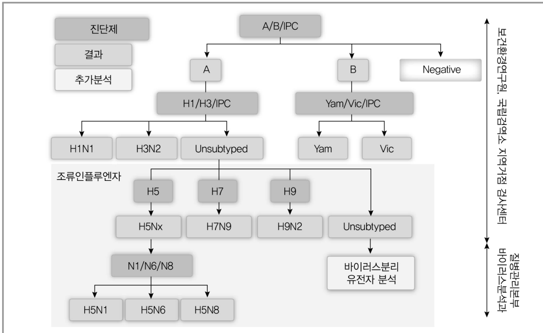
[그림] 인플루엔자 실험실 검사 체계도
