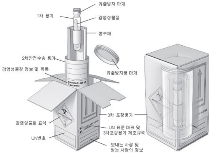
〈그림 23〉 카테고리 A 감염성물질 포장 방법(예시)
